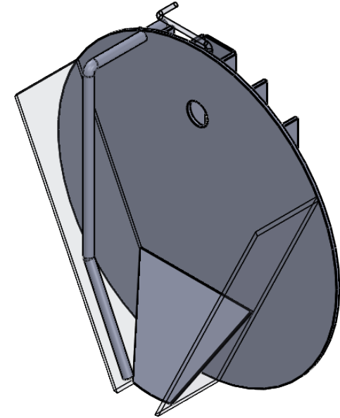
BIOPUHASTI PIPING SCALE 1:20
